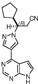
Ruxolitinib
