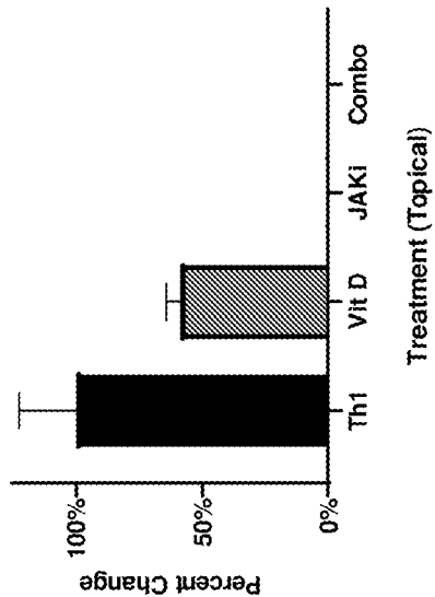
FIG. 9C Cxcl10
