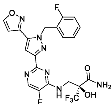
Formula IC
