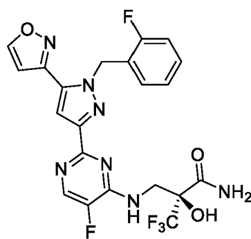
Formula IC
