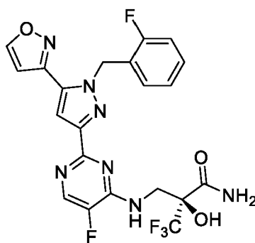
Formula IC
