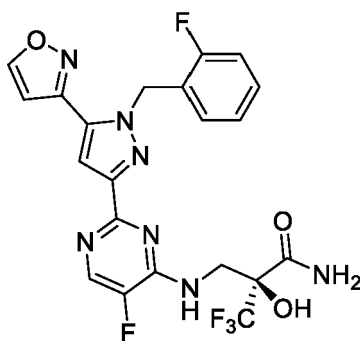
Formula IC
