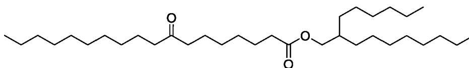
2-Hexyldecyl 8-oxooctadecanoate
