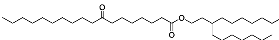
3-Heptyldecyl 8-oxooctadecanoate
