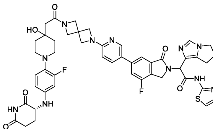
2-(6,7-dihydro-5H-pyrrolo[1,2-c]imidazol-1-yl)-2-(6-(6-(6-(2-(1-(4-(((R)-2,6-dioxopiperidin-3-yl)amino)-2-fluorophenyl)-4-hydroxypiperidin-4-yl)acetyl)-2,6-diazaspiro[3.3]heptan-2-yl)pyridin-3-yl)-4-fluoro-1-oxoisindolin-2-yl)-N-(thiazol-2-yl)acetamide
