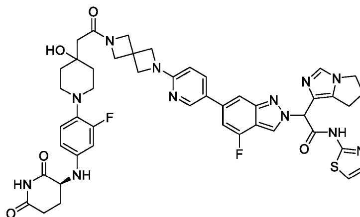
2-(6,7-dihydro-5H-pyrrolo[1,2-c]imidazol-1-yl)-2-(6-(6-(6-(2-(1-(4-(((S)-2,6-dioxopiperidin-3-yl)amino)-2-fluorophenyl)-4-hydroxypiperidin-4-yl)acetyl)-2,6-diazaspiro[3.3]heptan-2-yl)pyridin-3-yl)-4-fluoro-2H-indazol-2-yl)-N-(thiazol-2-yl)acetamide
