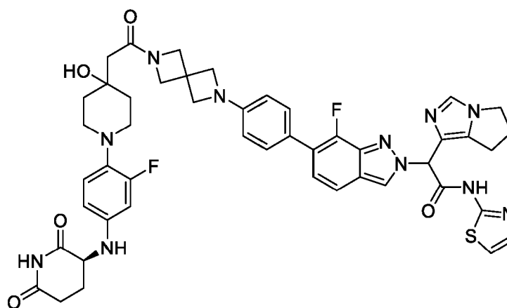
2-(6,7-dihydro-5H-pyrrolo[1,2-c]imidazol-1-yl)-2-(6-(4-(6-(2-(1-(4-(((S)-2,6-dioxopiperidin-3-yl)amino)-2-fluorophenyl)-4-hydroxypiperidin-4-yl)acetyl)-2,6-diazaspiro[3.3]heptan-2-yl)phenyl)-7-fluoro-2H-indazol-2-yl)-N-(thiazol-2-yl)acetamide
