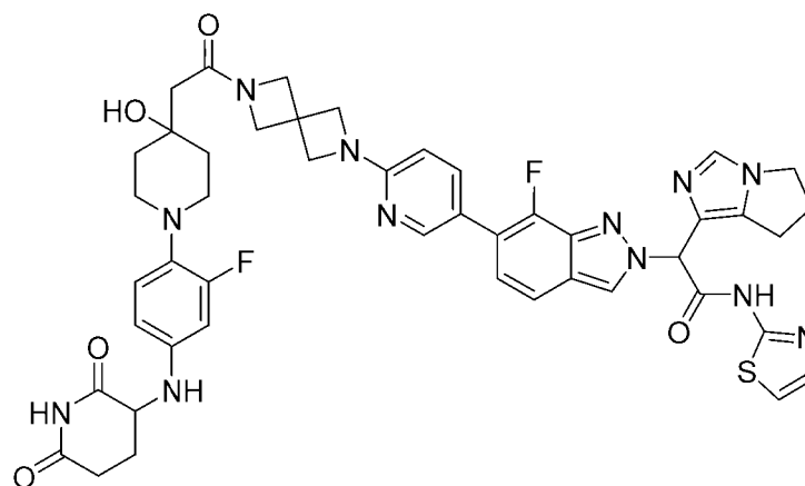
2-(6,7-dihydro-5H-pyrrolo[1,2-c]imidazol-1-yl)-2-(6-(6-(6-(2-(1-(4-((2,6-dioxopiperidin-3-yl)amino)-2-fluorophenyl)-4-hydroxypiperidin-4-yl)acetyl)-2,6-diazaspiro[3.3]heptan-2-yl)pyridin-3-yl)-7-fluoro-2H-indazol-2-yl)-N-(thiazol-2-yl)acetamide
