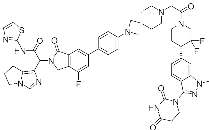
2-(6,7-dihydro-5H-pyrrolo[1,2-c]imidazol-1-yl)-2-(6-(4-(7-(2-((S)-4-(3-(2,4-dioxotetrahydropyrimidin-1(2H)-yl)-1-methyl-1H-indazol-6-yl)-3,3-difluoropiperidin-1-yl)-2-oxoethyl)-2,7-diazaspiro[3.5]nonan-2-yl)phenyl)-4-fluoro-1-oxoisindolin-2-yl)-N-(thiazol-2-yl)acetamide
