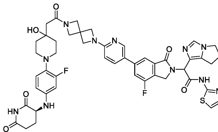
2-(6,7-dihydro-5H-pyrrolo[1,2-c]imidazol-1-yl)-2-(6-(6-(6-(2-(1-(4-(((S)-2,6-dioxopiperidin-3-yl)amino)-2-fluorophenyl)-4-hydroxypiperidin-4-yl)acetyl)-2,6-diazaspiro[3.3]heptan-2-yl)pyridin-3-yl)-4-fluoro-1-oxoisindolin-2-yl)-N-(thiazol-2-yl)acetamide
