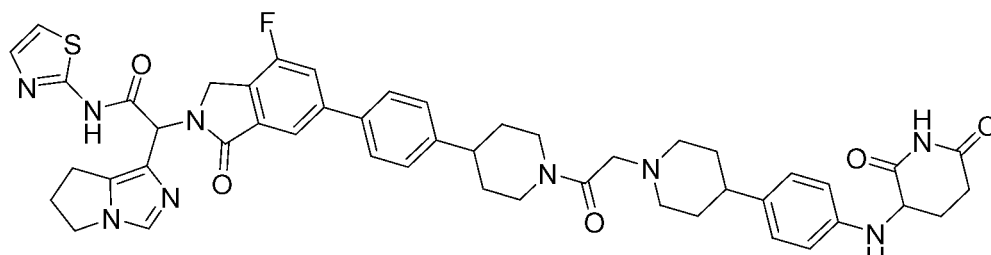
2-(6,7-dihydro-5H-pyrrolo[1,2-c]imidazol-1-yl)-2-(6-(4-(1-(2-(4-(4-((2,6-dioxopiperidin-3-yl)amino)phenyl)piperidin-1-yl)acetyl)piperidin-4-yl)phenyl)-4-fluoro-1-oxoisindolin-2-yl)-N-(thiazol-2-yl)acetamide
