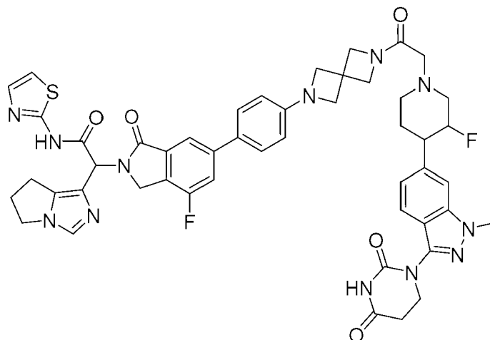
2-(6,7-dihydro-5H-pyrrolo[1,2-c]imidazol-1-yl)-2-(6-(4-(6-(2-(4-(3-(2,4-dioxotetrahydropyrimidin-1(2H)-yl)-1-methyl-1H-indazol-6-yl)-3-fluoropiperidin-1-yl)acetyl)-2,6-diazaspiro[3.3]heptan-2-yl)phenyl)-4-fluoro-1-oxoisindolin-2-yl)-N-(thiazol-2-yl)acetamide
