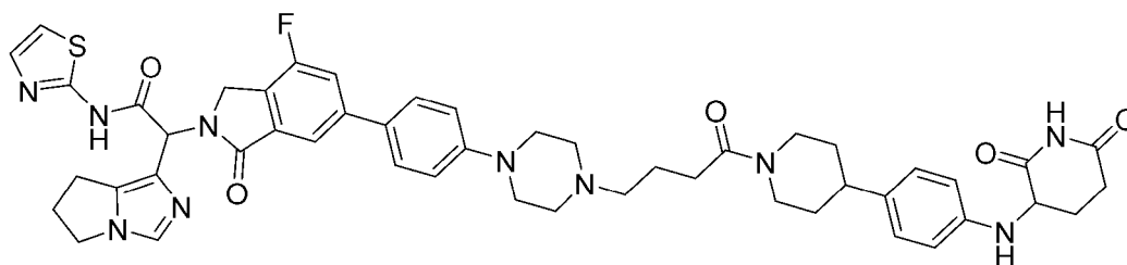
2-(6,7-dihydro-5H-pyrrolo[1,2-c]imidazol-1-yl)-2-(6-(4-(4-(4-(4-((2,6-dioxopiperidin-3-yl)amino)phenyl)piperidin-1-yl)-4-oxobutyl)piperazin-1-yl)phenyl)-4-fluoro-1-oxoisindolin-2-yl)-N-(thiazol-2-yl)acetamide
