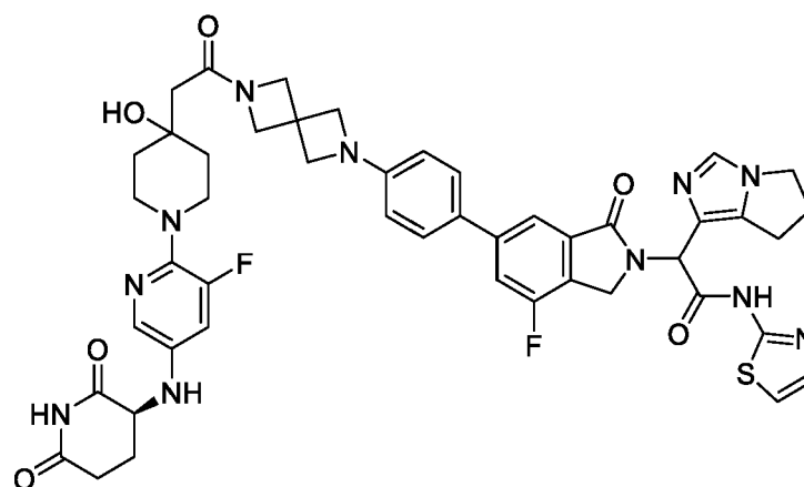
2-(6,7-dihydro-5H-pyrrolo[1,2-c]imidazol-1-yl)-2-(6-(4-(6-(2-(1-(5-(((S)-2,6-dioxopiperidin-3-yl)amino)-3-fluoropyridin-2-yl)-4-hydroxypiperidin-4-yl)acetyl)-2,6-diazaspiro[3.3]heptan-2-yl)phenyl)-4-fluoro-1-oxoisindolin-2-yl)-N-(thiazol-2-yl)acetamide
