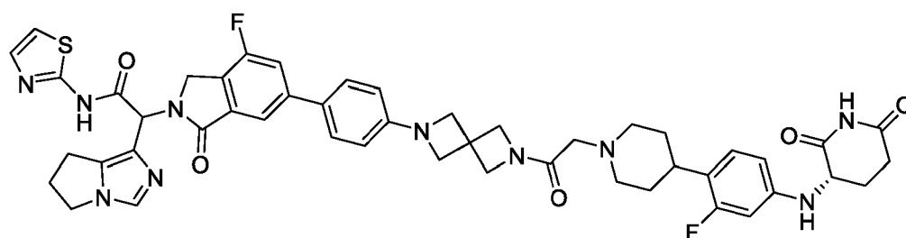
2-(6,7-dihydro-5H-pyrrolo[1,2-c]imidazol-1-yl)-2-[6-[4-[2-[2-[4-[4-[(3S)-2,6-dioxo-3-piperidyl]amino]-2-fluorophenyl]-1-piperidyl]acetyl]-2,6-diazaspiro[3.3]heptan-6-yl]phenyl]-4-fluoro-1-oxo-isoindolin-2-yl]-N-thiazol-2-yl-acetamide
