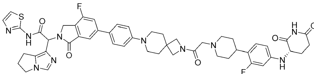
2-(6,7-dihydro-5H-pyrrolo[1,2-c]imidazol-1-yl)-2-(6-(4-(2-(2-(4-(4-(((S)-2,6-dioxopiperidin-3-yl)amino)-2-fluorophenyl)piperidin-1-yl)acetyl)-2,7-diazaspiro[3.5]nonan-7-yl)phenyl)-4-fluoro-1-oxoisindolin-2-yl)-N-(thiazol-2-yl)acetamide
