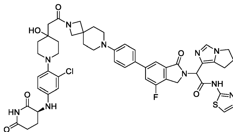
2-(6-(4-(2-(2-(1-(2-chloro-4-(((S)-2,6-dioxopiperidin-3-yl)amino)phenyl)-4-hydroxypiperidin-4-yl)acetyl)-2,7-diazaspiro[3.5]nonan-7-yl)phenyl)-4-fluoro-1-oxoisindolin-2-yl)-2-(6,7-dihydro-5H-pyrrolo[1,2-c]imidazol-1-yl)-N-(thiazol-2-yl)acetamide
