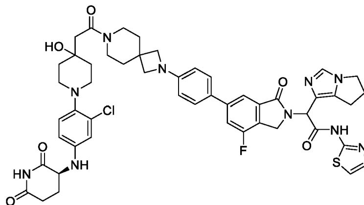
2-(6-(4-(7-(2-(1-(2-chloro-4-(((S)-2,6-dioxopiperidin-3-yl)amino)phenyl)-4-hydroxypiperidin-4-yl)acetyl)-2,7-diazaspiro[3.5]nonan-2-yl)phenyl)-4-fluoro-1-oxoisindolin-2-yl)-2-(6,7-dihydro-5H-pyrrolo[1,2-c]imidazol-1-yl)-N-(thiazol-2-yl)acetamide
