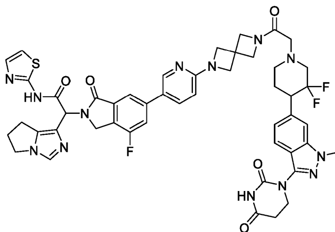
2-(6,7-dihydro-5H-pyrrolo[1,2-c]imidazol-1-yl)-2-(6-(6-(6-(2-(4-(3-(2,4-dioxotetrahydropyrimidin-1(2H)-yl)-1-methyl-1H-indazol-6-yl)-3,3-difluoropiperidin-1-yl)acetyl)-2,6-diazaspiro[3.3]heptan-2-yl)pyridin-3-yl)-4-fluoro-1-oxoisindolin-2-yl)-N-(thiazol-2-yl)acetamide
