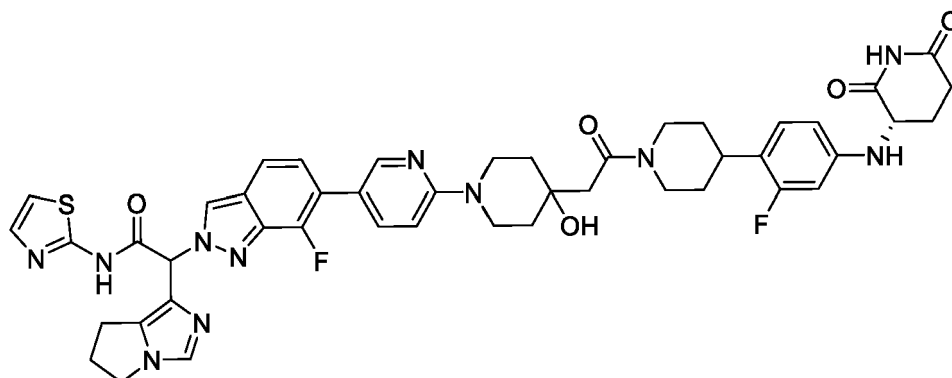
2-(6,7-dihydro-5H-pyrrolo[1,2-c]imidazol-1-yl)-2-[6-[6-[4-[2-[4-[4-[[[(3 S)-2,6-dioxo-3-piperidyl]amino]-2-fluoro-phenyl]-1-piperidyl]-2-oxo-ethyl]-4-hydroxy-1-piperidyl]-3-pyridyl]-7-fluoro-indazol-2-yl]-N-thiazol-2-yl]-acetamide
