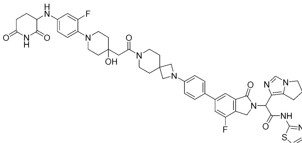
2-(6,7-dihydro-5H-pyrrolo[1,2-c]imidazol-1-yl)-2-(6-(4-(7-(2-(1-(4-((2,6-dioxopiperidin-3-yl)amino)-2-fluorophenyl)-4-hydroxypiperidin-4-yl)acetyl)-2,7-diazaspiro[3.5]nonan-2-yl)phenyl)-4-fluoro-1-oxoisindolin-2-yl)-N-(thiazol-2-yl)acetamide
