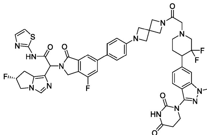
2-(6-(4-(6-(2-(4-(3-(2,4-dioxotetrahydropyrimidin-1(2H)-yl)-1-methyl-1H-indazol-6-yl)-3,3-difluoropiperidin-1-yl)acetyl)-2,6-diazaspiro[3.3]heptan-2-yl)phenyl)-4-fluoro-1-oxoisindolin-2-yl)-2-((R)-6-fluoro-6,7-dihydro-5H-pyrrolo[1,2-c]imidazol-1-yl)-N-(thiazol-2-yl)acetamide
