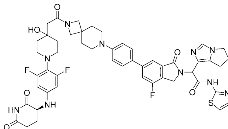
2-(6,7-dihydro-5H-pyrrolo[1,2-c]imidazol-1-yl)-2-(6-(4-(2-(2-(1-(4-(((S)-2,6-dioxopiperidin-3-yl)amino)-2,6-difluorophenyl)-4-hydroxypiperidin-4-yl)acetyl)-2,7-diazaspiro[3.5]nonan-7-yl)phenyl)-4-fluoro-1-oxoisindolin-2-yl)-N-(thiazol-2-yl)acetamide
