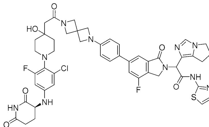
2-(6-(4-(6-(2-(1-(2-chloro-4-(((S)-2,6-dioxopiperidin-3-yl)amino)-6-fluorophenyl)-4-hydroxypiperidin-4-yl)acetyl)-2,6-diazaspiro[3.3]heptan-2-yl)phenyl)-4-fluoro-1-oxoisindolin-2-yl)-2-(6,7-dihydro-5H-pyrrolo[1,2-c]imidazol-1-yl)-N-(thiazol-2-yl)acetamide
