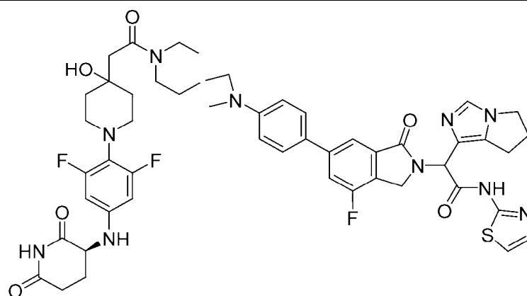
2-(6,7-dihydro-5H-pyrrolo[1,2-c]imidazol-1-yl)-2-(6-(4-(7-(2-(1-(4-(((S)-2,6-dioxopiperidin-3-yl)amino)-2,6-difluorophenyl)-4-hydroxypiperidin-4-yl)acetyl)-2,7-diazaspiro[3.5]nonan-2-yl)phenyl)-4-fluoro-1-oxoisindolin-2-yl)-N-(thiazol-2-yl)acetamide
