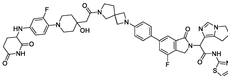
2-(6,7-dihydro-5H-pyrrolo[1,2-c]imidazol-1-yl)-2-(6-(4-(6-(2-(1-(4-((2,6-dioxopiperidin-3-yl)amino)-2-fluorophenyl)-4-hydroxypiperidin-4-yl)acetyl)-2,6-diazaspiro[3.4]octan-2-yl)phenyl)-4-fluoro-1-oxoisindolin-2-yl)-N-(thiazol-2-yl)acetamide
