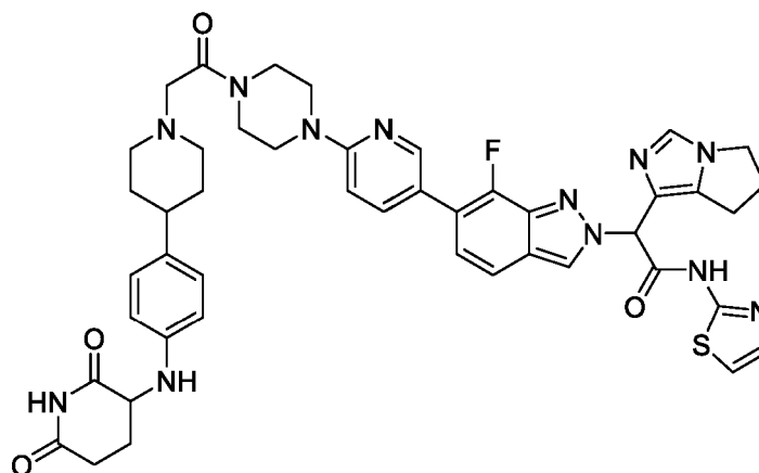
2-(6,7-dihydro-5H-pyrrolo[1,2-c]imidazol-1-yl)-2-(6-(6-(4-(2-(4-(4-((2,6-dioxopiperidin-3-yl)amino)phenyl)piperidin-1-yl)acetyl)piperazin-1-yl)pyridin-3-yl)-7-fluoro-2H-indazol-2-yl)-N-(thiazol-2-yl)acetamide
