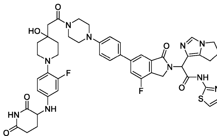
2-(6,7-dihydro-5H-pyrrolo[1,2-c]imidazol-1-yl)-2-(6-(4-(4-(2-(1-(4-((2,6-dioxopiperidin-3-yl)amino)-2-fluorophenyl)-4-hydroxypiperidin-4-yl)acetyl)piperazin-1-yl)phenyl)-4-fluoro-1-oxoisindolin-2-yl)-N-(thiazol-2-yl)acetamide
