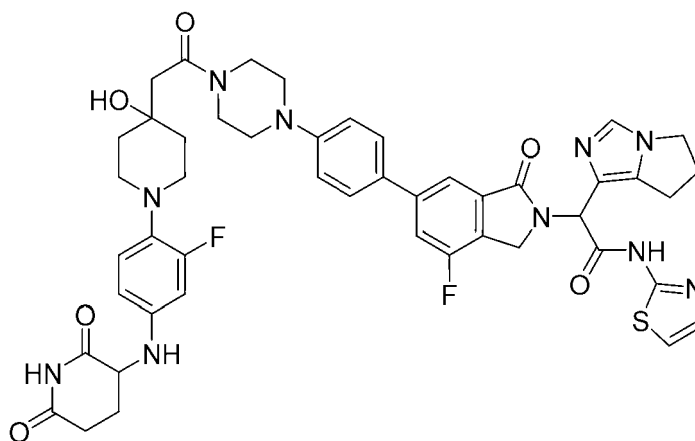
2-(6,7-dihydro-5H-pyrrolo[1,2-c]imidazol-1-yl)-2-(6-(4-(4-(2-(1-(4-((2,6-dioxopiperidin-3-yl)amino)-2-fluorophenyl)-4-hydroxypiperidin-4-yl)acetyl)piperazin-1-yl)phenyl)-4-fluoro-1-oxoisindolin-2-yl)-N-(thiazol-2-yl)acetamide
