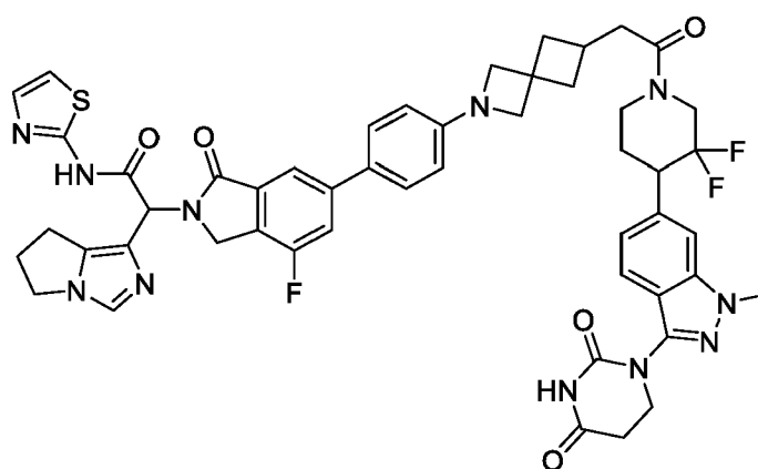
2-(6,7-dihydro-5H-pyrrolo[1,2-c]imidazol-1-yl)-2-(6-(4-(6-(2-(4-(3-(2,4-dioxotetrahydropyrimidin-1(2H)-yl)-1-methyl-1H-indazol-6-yl)-3,3-difluoropiperidin-1-yl)-2-oxoethyl)-2-azaspiro[3.3]heptan-2-yl)phenyl)-4-fluoro-1-oxoisindolin-2-yl)-N-(thiazol-2-yl)acetamide
