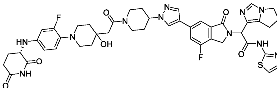
2-(6,7-dihydro-5H-pyrrolo[1,2-c]imidazol-1-yl)-2-(6-(1-(1-(2-(1-(4-(((S)-2,6-dioxopiperidin-3-yl)amino)-2-fluorophenyl)-4-hydroxypiperidin-4-yl)acetyl)piperidin-4-yl)-1H-pyrazol-4-yl)-4-fluoro-1-oxoisindolin-2-yl)-N-(thiazol-2-yl)acetamide
