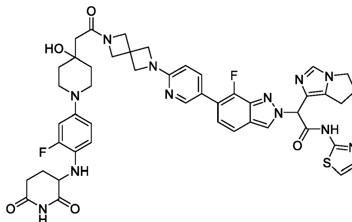
2-(6,7-dihydro-5H-pyrrolo[1,2-c]imidazol-1-yl)-2-(6-(6-(6-(2-(1-(4-((2,6-dioxopiperidin-3-yl)amino)-3-fluorophenyl)-4-hydroxypiperidin-4-yl)acetyl)-2,6-diazaspiro[3.3]heptan-2-yl)pyridin-3-yl)-7-fluoro-2H-indazol-2-yl)-N-(thiazol-2-yl)acetamide
