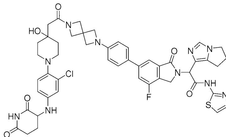
2-(6-(4-(6-(2-(1-(2-chloro-4-((2,6-dioxopiperidin-3-yl)amino)phenyl)-4-hydroxypiperidin-4-yl)acetyl)-2,6-diazaspiro[3.3]heptan-2-yl)phenyl)-4-fluoro-1-oxoisindolin-2-yl)-2-(6,7-dihydro-5H-pyrrolo[1,2-c]imidazol-1-yl)-N-(thiazol-2-yl)acetamide
