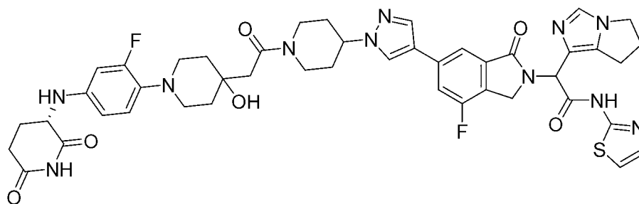
2-(6,7-dihydro-5H-pyrrolo[1,2-c]imidazol-1-yl)-2-(6-(1-(1-(2-(1-(4-(((S)-2,6-dioxopiperidin-3-yl)amino)-2-fluorophenyl)-4-hydroxypiperidin-4-yl)acetyl)piperidin-4-yl)-1H-pyrazol-4-yl)-4-fluoro-1-oxoisindolin-2-yl)-N-(thiazol-2-yl)acetamide
