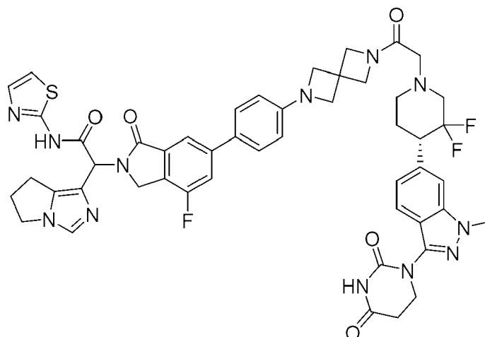
2-(6,7-dihydro-5H-pyrrolo[1,2-c]imidazol-1-yl)-2-(6-(4-(6-(2-((S)-4-(3-(2,4-dioxotetrahydropyrimidin-1(2H)-yl)-1-methyl-1H-indazol-6-yl)-3,3-difluoropiperidin-1-yl)acetyl)-2,6-diazaspiro[3.3]heptan-2-yl)phenyl)-4-fluoro-1-oxoisindolin-2-yl)-N-(thiazol-2-yl)acetamide
