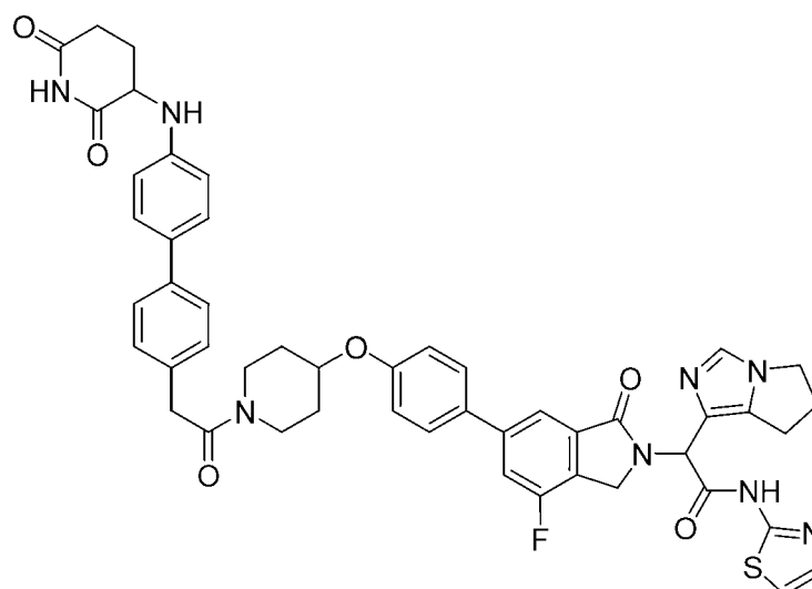
2-(6,7-dihydro-5H-pyrrolo[1,2-c]imidazol-1-yl)-2-(6-(4-((1-(2-(4'-((2,6-dioxopiperidin-3-yl)amino)-[1,1'-biphenyl]-4-yl)acetyl)piperidin-4-yl)oxy)phenyl)-4-fluoro-1-oxoisindolin-2-yl)-N-(thiazol-2-yl)acetamide
