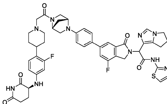
2-(6,7-dihydro-5H-pyrrolo[1,2-c]imidazol-1-yl)-2-(6-(4-((1R,4R)-5-(2-(4-(4-(((S)-2,6-dioxopiperidin-3-yl)amino)-2-fluorophenyl)piperidin-1-yl)acetyl)-2,5-diazabicyclo[2.2.1]heptan-2-yl)phenyl)-4-fluoro-1-oxoisindolin-2-yl)-N-(thiazol-2-yl)acetamide
