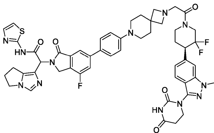
2-(6,7-dihydro-5H-pyrrolo[1,2-c]imidazol-1-yl)-2-(6-(4-(2-(2-((R)-4-(3-(2,4-dioxotetrahydropyrimidin-1(2H)-yl)-1-methyl-1H-indazol-6-yl)-3,3-difluoropiperidin-1-yl)-2-oxoethyl)-2,7-diazaspiro[3.5]nonan-7-yl)phenyl)-4-fluoro-1-oxoisindolin-2-yl)-N-(thiazol-2-yl)acetamide
