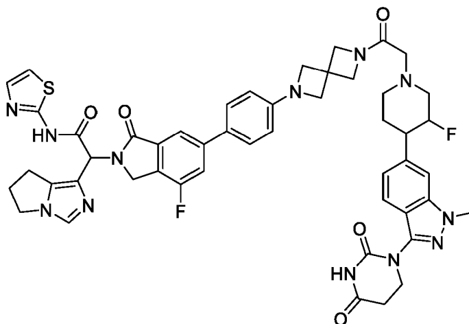
2-(6,7-dihydro-5H-pyrrolo[1,2-c]imidazol-1-yl)-2-(6-(4-(6-(2-(4-(3-(2,4-dioxotetrahydropyrimidin-1(2H)-yl)-1-methyl-1H-indazol-6-yl)-3-fluoropiperidin-1-yl)acetyl)-2,6-diazaspiro[3.3]heptan-2-yl)phenyl)-4-fluoro-1-oxoisindolin-2-yl)-N-(thiazol-2-yl)acetamide
