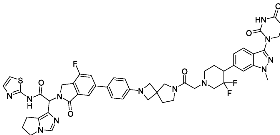
2-(6,7-dihydro-5H-pyrrolo[1,2-c]imidazol-1-yl)-2-(6-(4-(6-(2-(4-(3-(2,4-dioxotetrahydropyrimidin-1(2H)-yl)-1-methyl-1H-indazol-6-yl)-3,3-difluoropiperidin-1-yl)acetyl)-2,6-diazaspiro[3.4]octan-2-yl)phenyl)-4-fluoro-1-oxoisindolin-2-yl)-N-(thiazol-2-yl)acetamide
