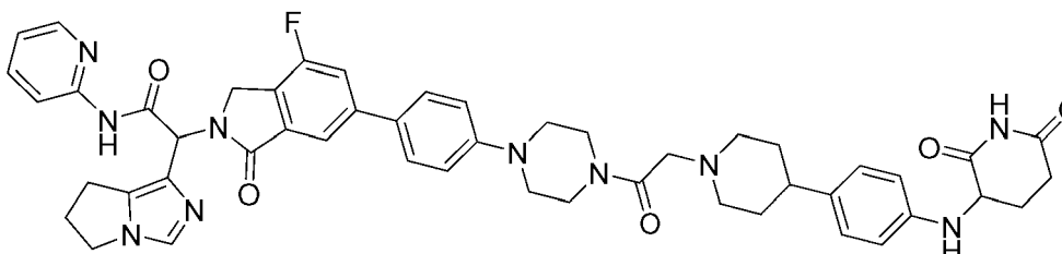
2-(6,7-dihydro-5H-pyrrolo[1,2-c]imidazol-1-yl)-2-(6-(4-(4-(2-(4-(4-((2,6-dioxopiperidin-3-yl)amino)phenyl)piperidin-1-yl)acetyl)piperazin-1-yl)phenyl)-4-fluoro-1-oxoisindolin-2-yl)-N-(pyridin-2-yl)acetamide
