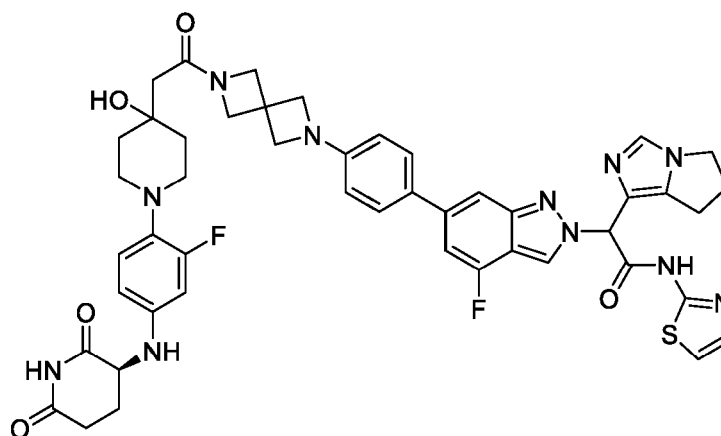
2-(6,7-dihydro-5H-pyrrolo[1,2-c]imidazol-1-yl)-2-(6-(4-(6-(2-(1-(4-(((S)-2,6-dioxopiperidin-3-yl)amino)-2-fluorophenyl)-4-hydroxypiperidin-4-yl)acetyl)-2,6-diazaspiro[3.3]heptan-2-yl)phenyl)-4-fluoro-2H-indazol-2-yl)-N-(thiazol-2-yl)acetamide
