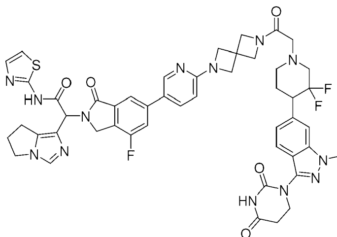
2-(6,7-dihydro-5H-pyrrolo[1,2-c]imidazol-1-yl)-2-(6-(6-(6-(2-(4-(3-(2,4-dioxotetrahydropyrimidin-1(2H)-yl)-1-methyl-1H-indazol-6-yl)-3,3-difluoropiperidin-1-yl)acetyl)-2,6-diazaspiro[3.3]heptan-2-yl)pyridin-3-yl)-4-fluoro-1-oxoisindolin-2-yl)-N-(thiazol-2-yl)acetamide
