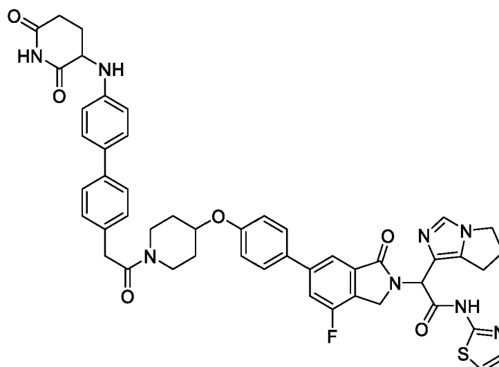
2-(6,7-dihydro-5H-pyrrolo[1,2-c]imidazol-1-yl)-2-(6-(4-((1-(2-(4'-((2,6-dioxopiperidin-3-yl)amino)-[1,1'-biphenyl]-4-yl)acetyl)piperidin-4-yl)oxy)phenyl)-4-fluoro-1-oxoisindolin-2-yl)-N-(thiazol-2-yl)acetamide
