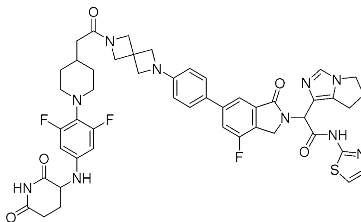
2-(6,7-dihydro-5H-pyrrolo[1,2-c]imidazol-1-yl)-2-(6-(4-(6-(2-(1-(4-((2,6-dioxopiperidin-3-yl)amino)-2,6-difluorophenyl)piperidin-4-yl)acetyl)-2,6-diazaspiro[3.3]heptan-2-yl)phenyl)-4-fluoro-1-oxoisindolin-2-yl)-N-(thiazol-2-yl)acetamide
