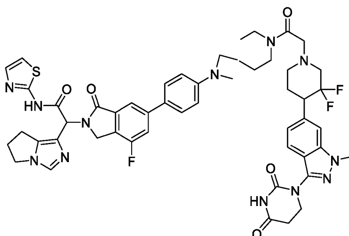
2-(6,7-dihydro-5H-pyrrolo[1,2-c]imidazol-1-yl)-2-(6-(4-(7-(2-(4-(3-(2,4-dioxotetrahydropyrimidin-1(2H)-yl)-1-methyl-1H-indazol-6-yl)-3,3-difluoropiperidin-1-yl)acetyl)-2,7-diazaspiro[3.5]nonan-2-yl)phenyl)-4-fluoro-1-oxoisindolin-2-yl)-N-(thiazol-2-yl)acetamide
