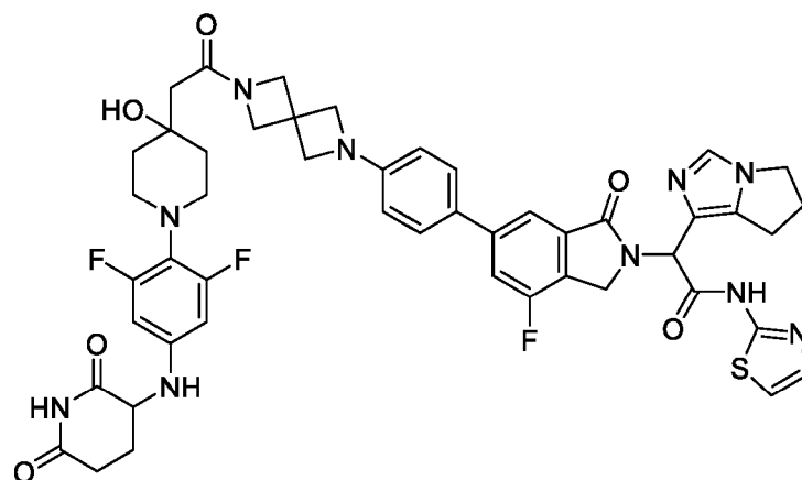
2-(6,7-dihydro-5H-pyrrolo[1,2-c]imidazol-1-yl)-2-(6-(4-(6-(2-(1-(4-((2,6-dioxopiperidin-3-yl)amino)-2,6-difluorophenyl)-4-hydroxypiperidin-4-yl)acetyl)-2,6-diazaspiro[3.3]heptan-2-yl)phenyl)-4-fluoro-1-oxoisindolin-2-yl)-N-(thiazol-2-yl)acetamide
