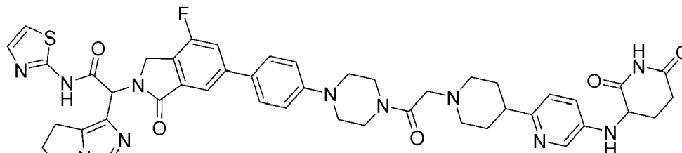
2-(6,7-dihydro-5H-pyrrolo[1,2-c]imidazol-1-yl)-2-[6-[4-[4-[2-[4-[5-[(2,6-dioxo-3-piperidyl)amino]-2-pyridyl]-1-piperidyl]acetyl]piperazin-1-yl]phenyl]-4-fluoro-1-oxo-isindolin-2-yl]-N-thiazol-2-yl-acetamide
