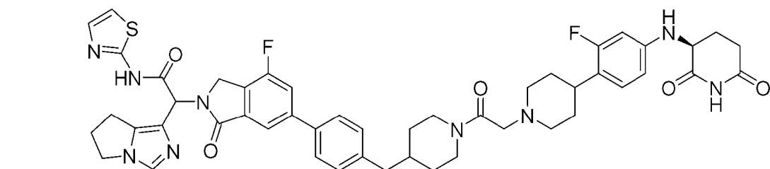
2-(6,7-dihydro-5H-pyrrolo[1,2-c]imidazol-1-yl)-2-[6-[4-[[1-[2-[4-[4-[[[(3S)-2,6-dioxo-3-piperidyl]amino]-2-fluoro-phenyl]-1-piperidyl]acetyl]-4-piperidyl]methyl]phenyl]-4-fluoro-1-oxo-isoindolin-2-yl]-N-thiazol-2-yl]-acetamide
