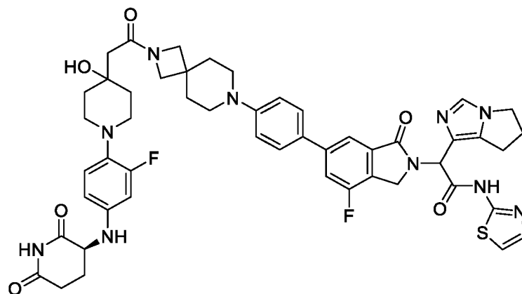
2-(6,7-dihydro-5H-pyrrolo[1,2-c]imidazol-1-yl)-2-(6-(4-(2-(2-(1-(4-(((S)-2,6-dioxopiperidin-3-yl)amino)-2-fluorophenyl)-4-hydroxypiperidin-4-yl)acetyl)-2,7-diazaspiro[3.5]nonan-7-yl)phenyl)-4-fluoro-1-oxoisindolin-2-yl)-N-(thiazol-2-yl)acetamide
