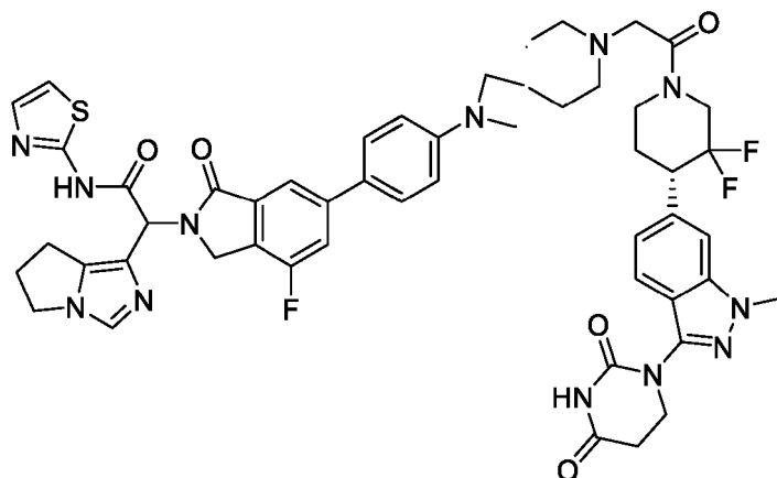
2-(6,7-dihydro-5H-pyrrolo[1,2-c]imidazol-1-yl)-2-(6-(4-(7-(2-((S)-4-(3-(2,4-dioxotetrahydropyrimidin-1(2H)-yl)-1-methyl-1H-indazol-6-yl)-3,3-difluoropiperidin-1-yl)-2-oxoethyl)-2,7-diazaspiro[3.5]nonan-2-yl)phenyl)-4-fluoro-1-oxoisindolin-2-yl)-N-(thiazol-2-yl)acetamide
