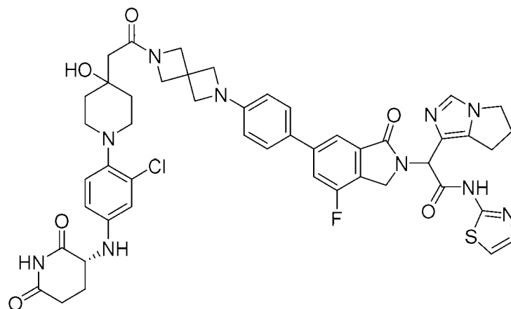
2-(6-(4-(6-(2-(1-(2-chloro-4-(((R)-2,6-dioxopiperidin-3-yl)amino)phenyl)-4-hydroxypiperidin-4-yl)acetyl)-2,6-diazaspiro[3.3]heptan-2-yl)phenyl)-4-fluoro-1-oxoisindolin-2-yl)-2-(6,7-dihydro-5H-pyrrolo[1,2-c]imidazol-1-yl)-N-(thiazol-2-yl)acetamide
