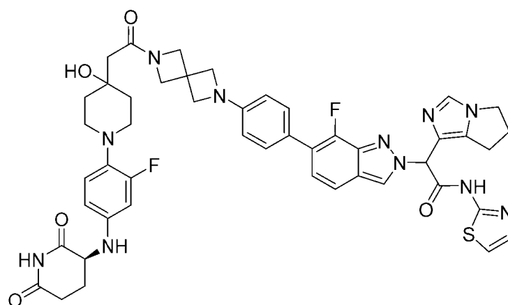
2-(6,7-dihydro-5H-pyrrolo[1,2-c]imidazol-1-yl)-2-(6-(4-(6-(2-(1-(4-(((S)-2,6-dioxopiperidin-3-yl)amino)-2-fluorophenyl)-4-hydroxypiperidin-4-yl)acetyl)-2,6-diazaspiro[3.3]heptan-2-yl)phenyl)-7-fluoro-2H-indazol-2-yl)-N-(thiazol-2-yl)acetamide
