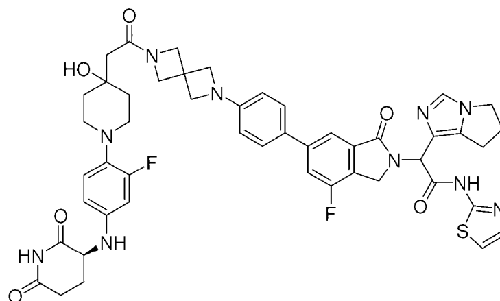
7-dihydro-5H-pyrrolo[1,2-c]imidazol-1-yl)-2-(6-(4-(6-(2-(1-(4-(((S)-2-(6,2,6-dioxopiperidin-3-yl)amino)-2-fluorophenyl)-4-hydroxypiperidin-4-yl)acetyl)-2,6-diazaspiro[3.3]heptan-2-yl)phenyl)-4-fluoro-1-oxoisindolin-2-yl)-N-(thiazol-2-yl)acetamide
