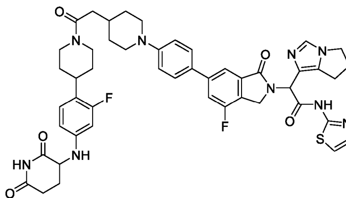
2-(6,7-dihydro-5H-pyrrolo[1,2-c]imidazol-1-yl)-2-(6-(4-(4-(2-(4-(4-((2,6-dioxopiperidin-3-yl)amino)-2-fluorophenyl)piperidin-1-yl)-2-oxoethyl)piperidin-1-yl)phenyl)-4-fluoro-1-oxoisindolin-2-yl)-N-(thiazol-2-yl)acetamide
