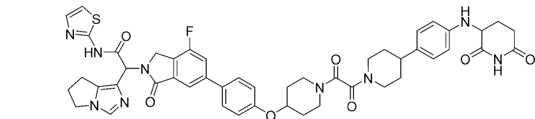
2-(6,7-dihydro-5H-pyrrolo[1,2-c]imidazol-1-yl)-2-[6-[4-[[1-[2-[4-[4-[(2,6-dioxo-3-piperidyl)amino]phenyl]-1-piperidyl]-2-oxo-acetyl]-4-piperidyl]oxy]phenyl]-4-fluoro-1-oxo-isindolin-2-yl]-N-thiazol-2-yl-acetamide
