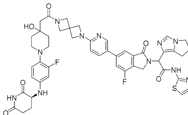
2-(6,7-dihydro-5H-pyrrolo[1,2-c]imidazol-1-yl)-2-(6-(6-(6-(2-(1-(4-(((S)-2,6-dioxopiperidin-3-yl)amino)-2-fluorophe-nyl)-4-hydroxypiperidin-4-yl)acetyl)-2,6-diazaspiro[3.3]heptan-2-yl)pyridin-3-yl)-4-fluoro-1-oxoisindolin-2-yl)-N-(thiazol-2-yl)acetamide
