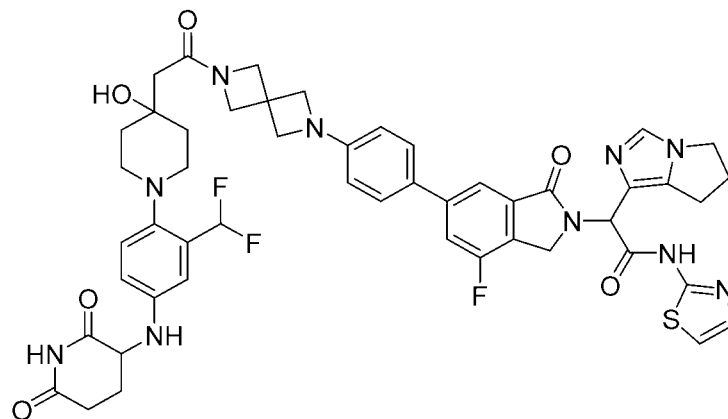
2-(6-(4-(6-(2-(1-(2-(difluoromethyl)-4-((2,6-dioxopiperidin-3-yl)amino)phenyl)-4-hydroxypiperidin-4-yl)acetyl)-2,6-diazaspiro[3.3]heptan-2-yl)phenyl)-4-fluoro-1-oxoisindolin-2-yl)-2-(6,7-dihydro-5H-pyrrolo[1,2-c]imidazol-1-yl)-N-(thiazol-2-yl)acetamide
