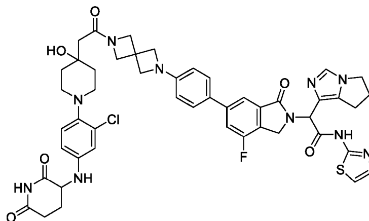
2-(6-(4-(6-(2-(1-(2-chloro-4-((2,6-dioxopiperidin-3-yl)amino)phenyl)-4-hydroxypiperidin-4-yl)acetyl)-2,6-diazaspiro[3.3]heptan-2-yl)phenyl)-4-fluoro-1-oxoisindolin-2-yl)-2-(6,7-dihydro-5H-pyrrolo[1,2-c]imidazol-1-yl)-N-(thiazol-2-yl)acetamide
