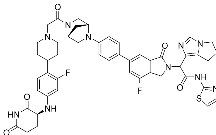
2-(6,7-dihydro-5H-pyrrolo[1,2-c]imidazol-1-yl)-2-(6-(4-((1R,4R)-5-(2-(4-(4-(((S)-2,6-dioxopiperidin-3-yl)amino)-2-fluorophenyl)piperidin-1-yl)acetyl)-2,5-diazabicyclo[2.2.1]heptan-2-yl)phenyl)-4-fluoro-1-oxoisindolin-2-yl)-N-(thiazol-2-yl)acetamide
