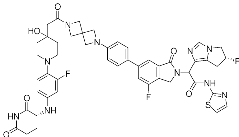
2-(6-(4-(6-(2-(1-(4-(((R)-2,6-dioxopiperidin-3-yl)amino)-2-fluorophenyl)-4-hydroxypiperidin-4-yl)acetyl)-2,6-diazaspiro[3.3]heptan-2-yl)phenyl)-4-fluoro-1-oxoisindolin-2-yl)-2-((R)-6-fluoro-6,7-dihydro-5H-pyrrolo[1,2-c]imidazol-1-yl)-N-(thiazol-2-yl)acetamide
