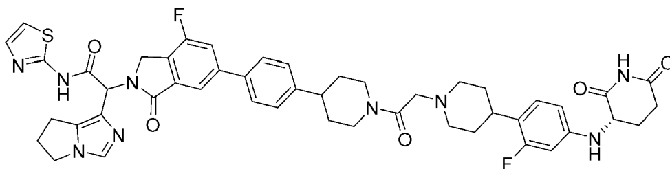
2-(6,7-dihydro-5H-pyrrolo[1,2-c]imidazol-1-yl)-2-(6-(4-(1-(2-(4-(4-(((S)-2,6-dioxopiperidin-3-yl)amino)-2-fluorophenyl)piperidin-1-yl)acetyl)piperidin-4-yl)phenyl)-4-fluoro-1-oxoisindolin-2-yl)-N-(thiazol-2-yl)acetamide
