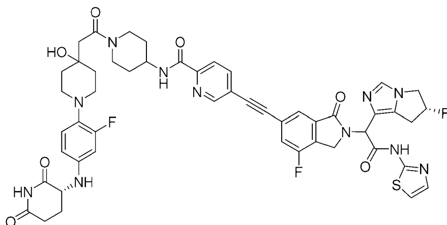
N-(1-(2-(1-(4-(((R)-2,6-dioxopiperidin-3-yl)amino)-2-fluorophenyl)-4-hydroxypiperidin-4-yl)acetyl)piperidin-4-yl)-5-((7-fluoro-2-(1-((R)-6-fluoro-6,7-dihydro-5H-pyrrolo[1,2-c]imidazol-1-yl)-2-oxo-2-(thiazol-2-ylamino)ethyl)-3-oxoisindolin-5-yl)ethynyl)picolinamide
