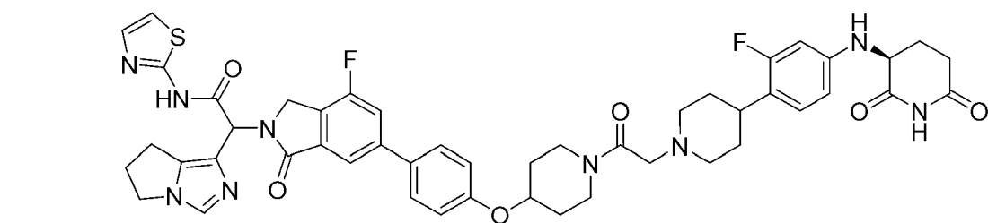
2-(6,7-dihydro-5H-pyrrolo[1,2-c]imidazol-1-yl)-2-(6-(4-((1-(2-(4-(4-(((S)-2,6-dioxopiperidin-3-yl)amino)-2-fluorophenyl)piperidin-1-yl)acetyl)piperidin-4-yl)oxy)phenyl)-4-fluoro-1-oxoisindolin-2-yl)-N-(thiazol-2-yl)acetamide
