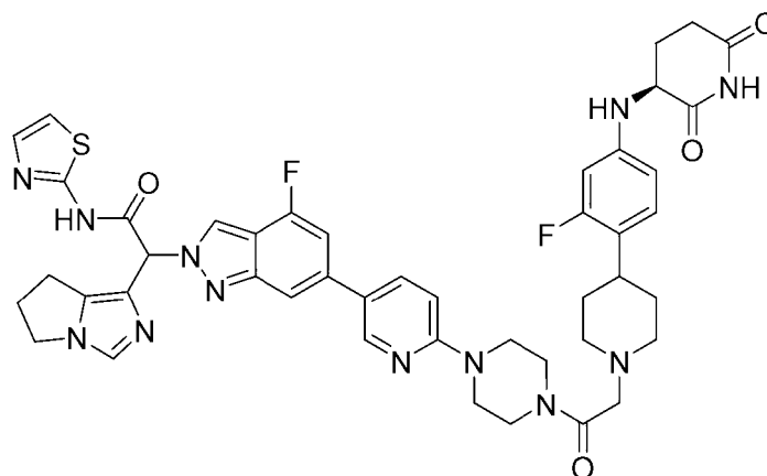
2-(6,7-dihydro-5H-pyrrolo[1,2-c]imidazol-1-yl)-2-(6-(6-(4-(2-(4-(4-(((S)-2,6-dioxopiperidin-3-yl)amino)-2-fluorophenyl)piperidin-1-yl)acetyl)piperazin-1-yl)pyridin-3-yl)-4-fluoro-2H-indazol-2-yl)-N-(thiazol-2-yl)acetamide
