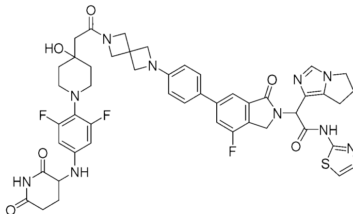
2-(6,7-dihydro-5H-pyrrolo[1,2-c]imidazol-1-yl)-2-(6-(4-(6-(2-(1-(4-((2,6-dioxopiperidin-3-yl)amino)-2,6-difluorophenyl)-4-hydroxypiperidin-4-yl)acetyl)-2,6-diazaspiro[3.3]heptan-2-yl)phenyl)-4-fluoro-1-oxoisindolin-2-yl)-N-(thiazol-2-yl)acetamide
