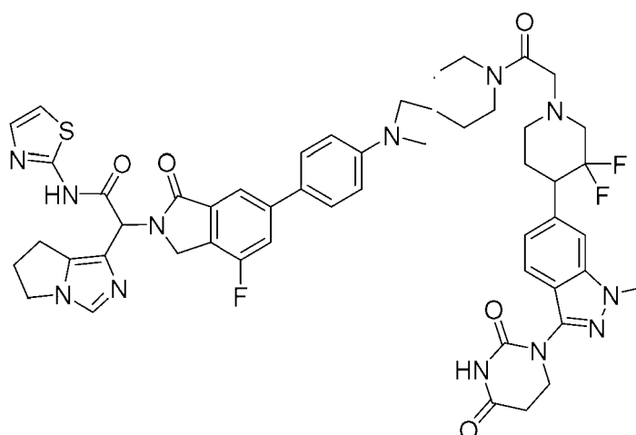
2-(6,7-dihydro-5H-pyrrolo[1,2-c]imidazol-1-yl)-2-(6-(4-(7-(2-(4-(3-(2,4-dioxotetrahydropyrimidin-1(2H)-yl)-1-methyl-1H-indazol-6-yl)-3,3-difluoropiperidin-1-yl)acetyl)-2,7-diazaspiro[3.5]nonan-2-yl)phenyl)-4-fluoro-1-oxoisindolin-2-yl)-N-(thiazol-2-yl)acetamide
