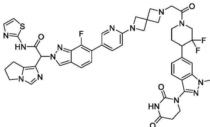
2-(6,7-dihydro-5H-pyrrolo[1,2-c]imidazol-1-yl)-2-(6-(6-(6-(2-(4-(3-(2,4-dioxotetrahydropyrimidin-1(2H)-yl)-1-methyl-1H-indazol-6-yl)-3,3-difluoropiperidin-1-yl)-2-oxoethyl)-2,6-diazaspiro[3.3]heptan-2-yl)pyridin-3-yl)-7-fluoro-2H-indazol-2-yl)-N-(thiazol-2-yl)acetamide
