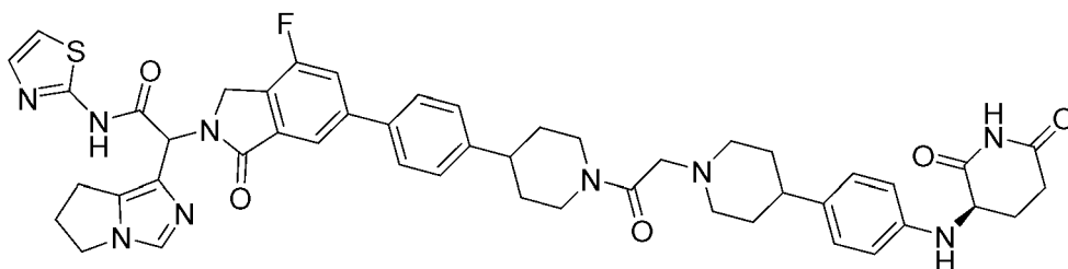
2-(6,7-dihydro-5H-pyrrolo[1,2-c]imidazol-1-yl)-2-(6-(4-(1-(2-(4-(4-(((R)-2,6-dioxopiperidin-3-yl)amino)phenyl)piperidin-1-yl)acetyl)piperidin-4-yl)phenyl)-4-fluoro-1-oxoisindolin-2-yl)-N-(thiazol-2-yl)acetamide
