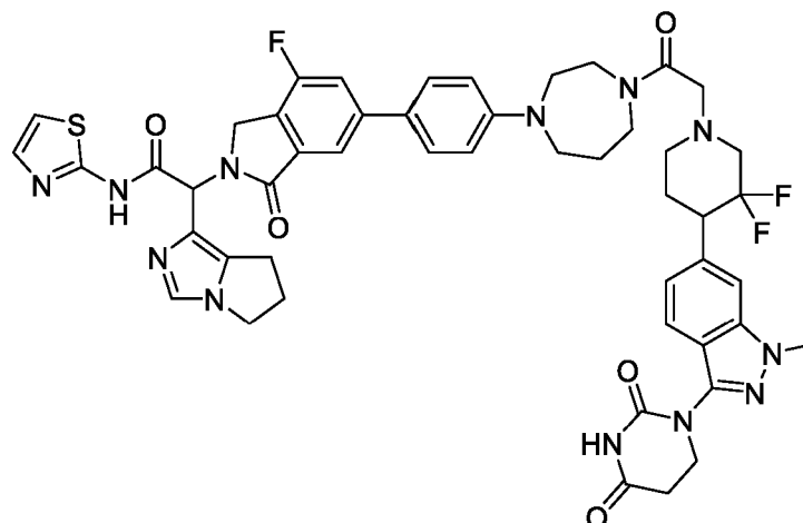
2-(6,7-dihydro-5H-pyrrolo[1,2-c]imidazol-1-yl)-2-(6-(4-(4-(2-(4-(3-(2,4-dioxotetrahydropyrimidin-1(2H)-yl)-1-methyl-1H-indazol-6-yl)-3,3-difluoropiperidin-1-yl)acetyl)-1,4-diazepan-1-yl)phenyl)-4-fluoro-1-oxoisindolin-2-yl)-N-(thiazol-2-yl)acetamide
