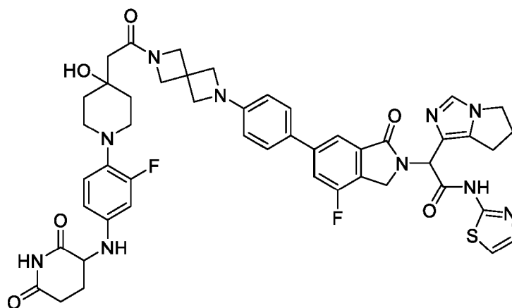
2-(6,7-dihydro-5H-pyrrolo[1,2-c]imidazol-1-yl)-2-(6-(4-(6-(2-(1-(4-((2,6-dioxopiperidin-3-yl)amino)-2-fluorophenyl)-4-hydroxypiperidin-4-yl)acetyl)-2,6-diazaspiro[3.3]heptan-2-yl)phenyl)-4-fluoro-1-oxoisindolin-2-yl)-N-(thiazol-2-yl)acetamide
