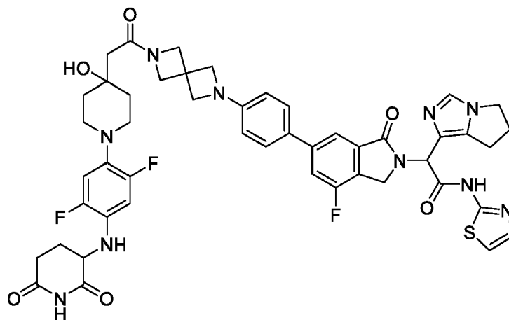
2-(6,7-dihydro-5H-pyrrolo[1,2-c]imidazol-1-yl)-2-(6-(4-(6-(2-(1-(4-((2,6-dioxopiperidin-3-yl)amino)-2,5-difluorophenyl)-4-hydroxypiperidin-4-yl)acetyl)-2,6-diazaspiro[3.3]heptan-2-yl)phenyl)-4-fluoro-1-oxoisindolin-2-yl)-N-(thiazol-2-yl)acetamide
