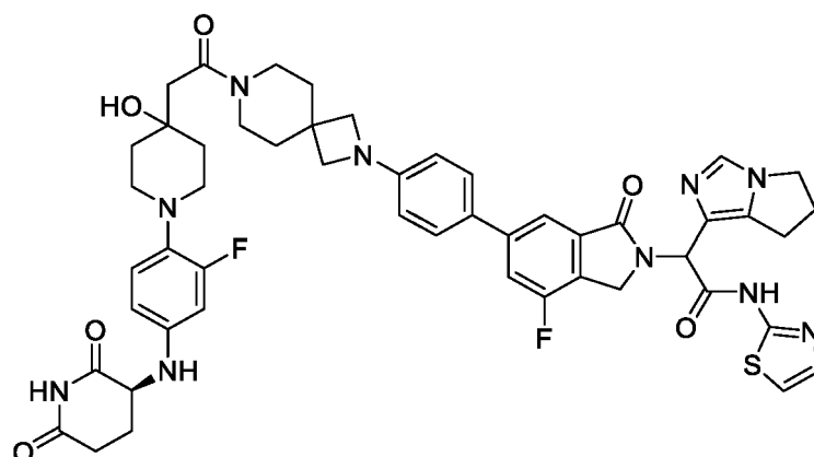
2-(6,7-dihydro-5H-pyrrolo[1,2-c]imidazol-1-yl)-2-(6-(4-(7-(2-(1-(4-(((S)-2,6-dioxopiperidin-3-yl)amino)-2-fluorophenyl)-4-hydroxypiperidin-4-yl)acetyl)-2,7-diazaspiro[3.5]nonan-2-yl)phenyl)-4-fluoro-1-oxoisindolin-2-yl)-N-(thiazol-2-yl)acetamide
