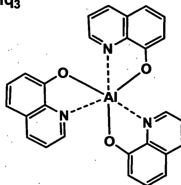
Alq 3
