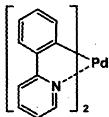
Pd-1
