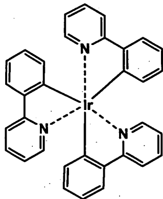
Ir-1
