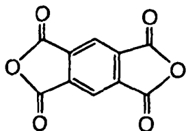
COMPOUND (d)
