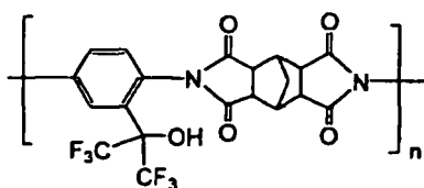
POLYMER (J)
