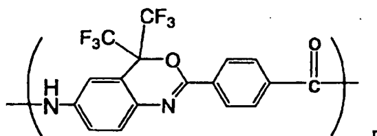
POLYMER (D)
