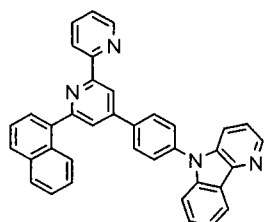
[Chem. 25]
