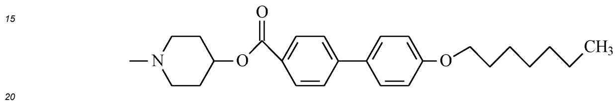
L(30a) 1-méthyl-4-((4'-(((1-méthylpipéridin-4-yl)oxy)carbonyl)-[1,1'-biphényl]-4-carbonyl)oxy)pipéridin-1-yle
