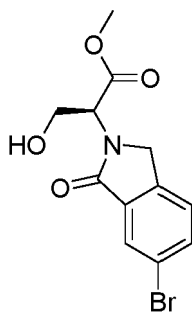
Methyl (S)-2-(6-bromo-1-oxoisindolin-2-yl)-3-hydroxypropanoate
