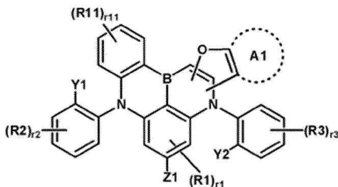
[Formule chimique 1-1]
