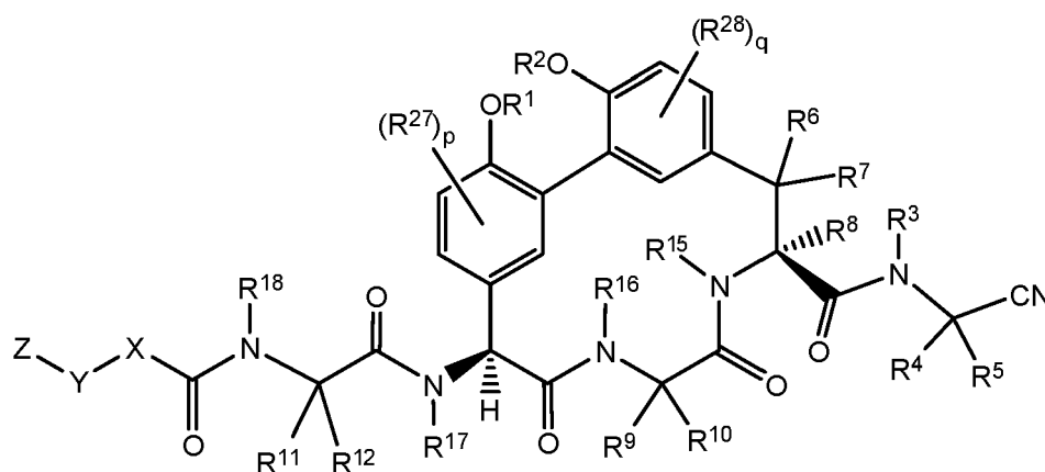
Formula (IVa);
