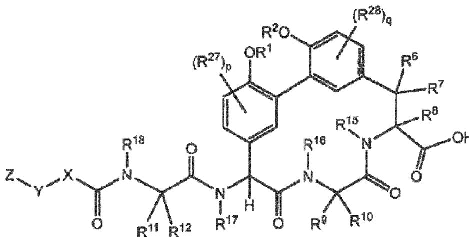
Formel (V);
