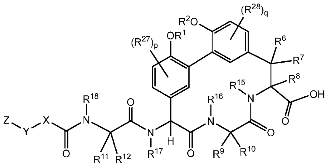
Formule (V) ;
