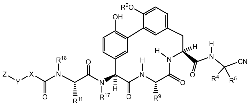
Formula (Ie);
