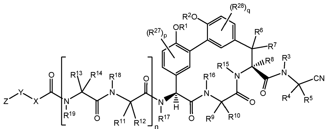
Formula (IIa);
